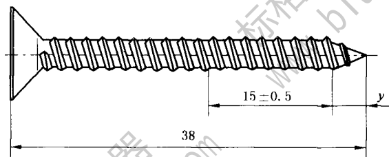
图 28 自攻螺钉
