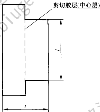
图 23 胶层剪切强度试件图
