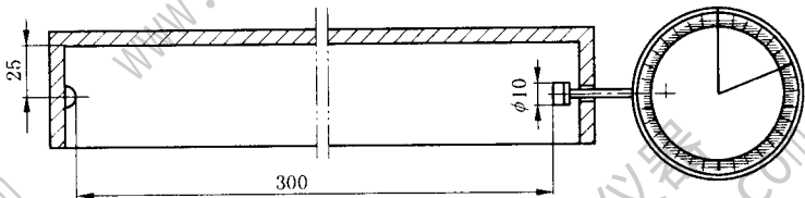
图 36 长度测量仪示例
