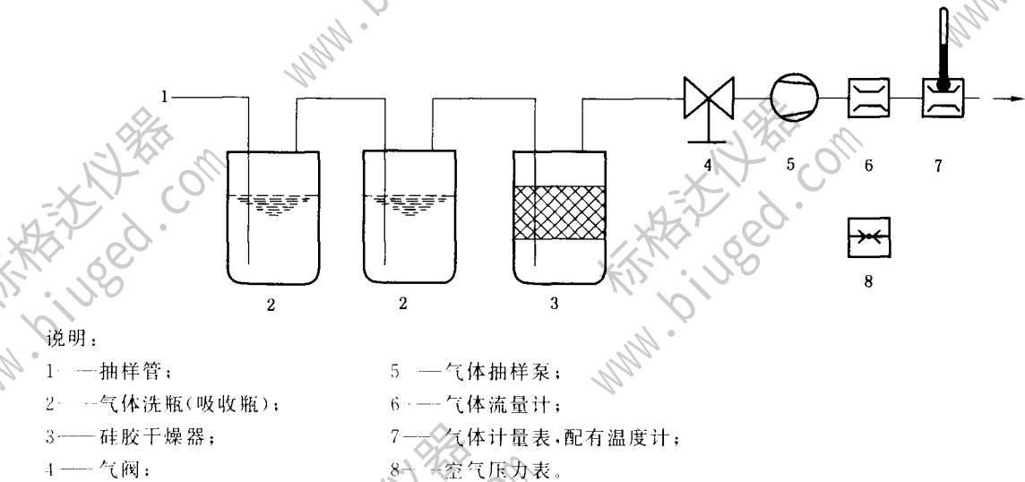
图 64 取样装置示例
