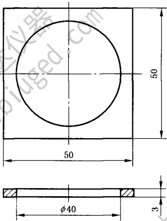
图 17 钢垫片(用于试件厚度 t \leq 10\text{ mm} )
