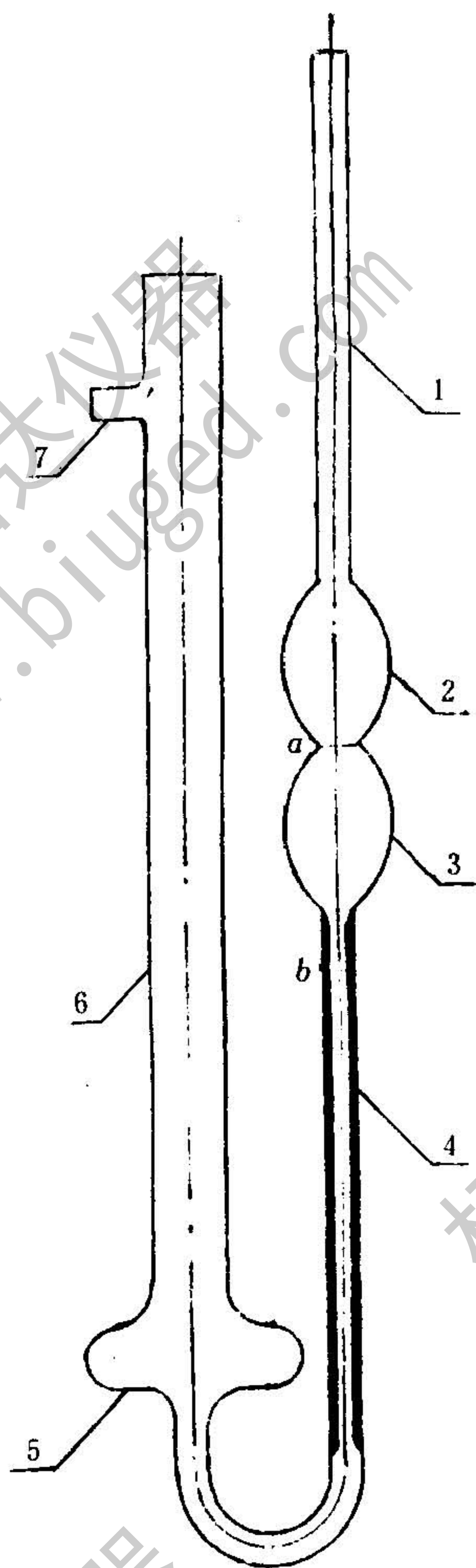
毛细管粘度计图
