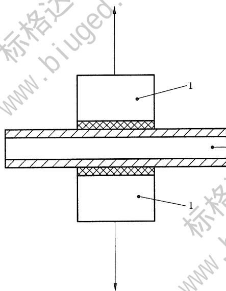
图 4 在单面或双面涂漆的底材上进行夹层式试验的试验组合
