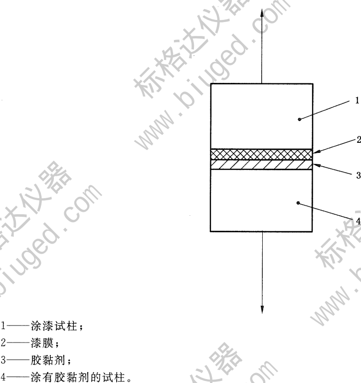
图 6 仅使用试柱的试验组合
