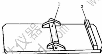
图 1 I 型弯曲试验仪示意图
