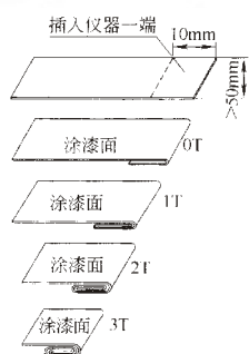
T弯试验示意图
